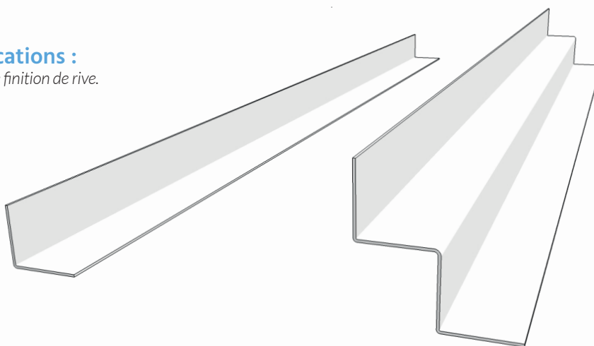
Cornière L de section droite : 19/24 mm
